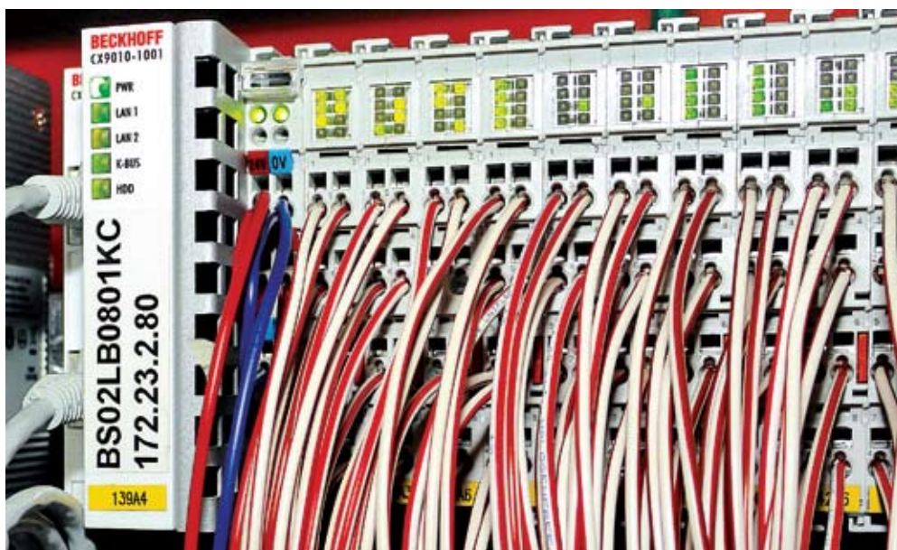
Рис.2 Сигналы, поступающие на датчики и исполнительные механизмы и идущие обратно, передаются с помощью модулей ввода/вывода Beckhoff и обрабатываются контроллером CX9010. Взаимодействие между системой, другими подстанциями и программной системой диспетчерского управления и сбора данных (SCADA) осуществляется через Ethernet с использованием оптоволоконных кабелей.
